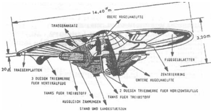
(Abb. 2.3.5: Risszeichnung des Schriever-Flugkreisels)
