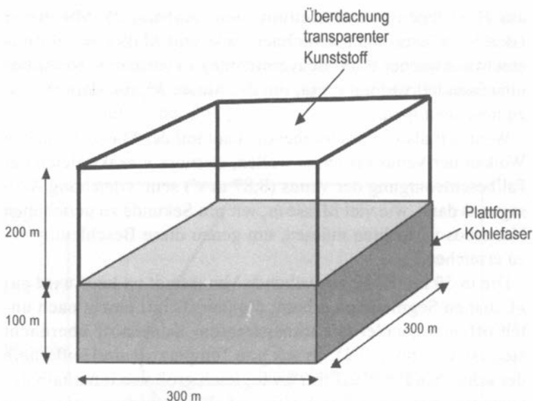
Abbildung 2.9.2: Schematische Darstellung eines Urbanen Segments.
