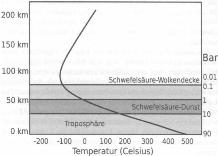
(Abb. 2.9.1: Temperatur und Druck auf der Venus als Funktion der Höhe 48 )
