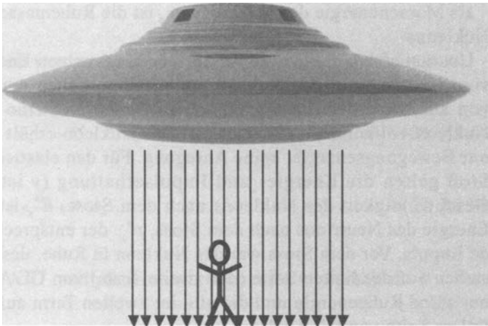
(Abb. A3.1: Neutrinofluss einer Flugscheibe)
