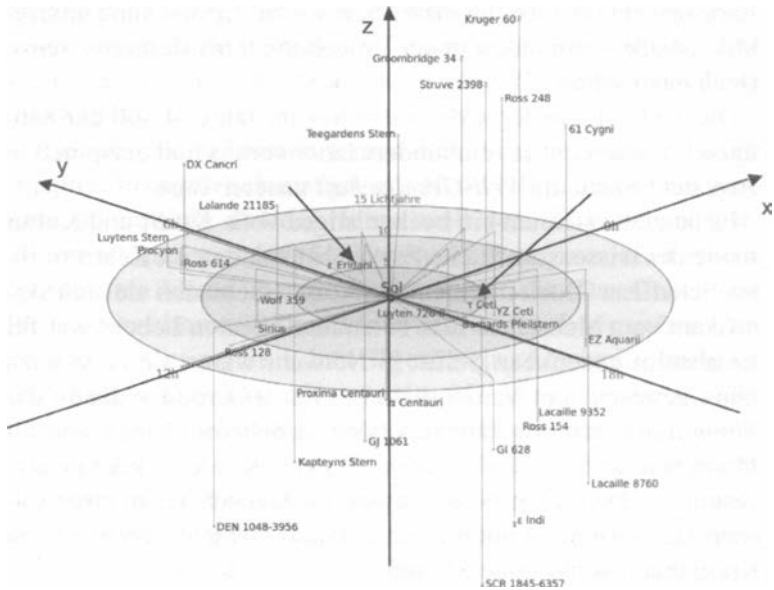
(Abb. 3.1.1: Räumliche Anordnung der Sterne in unserer kosmischen Nachbarschaft)
